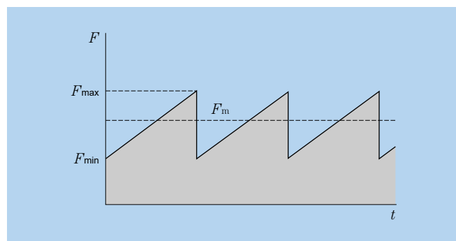
Fig. 4.10 Carga linear flutuante
