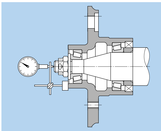
Fig. 15.13 Medição do ajuste da folga interna axial
