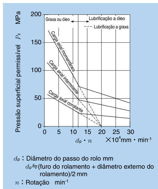
Fig. 1 Pressão superficial permissível do flange
