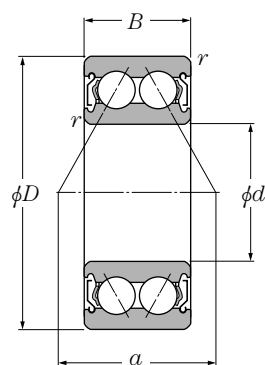
Blindado (ZZ)
