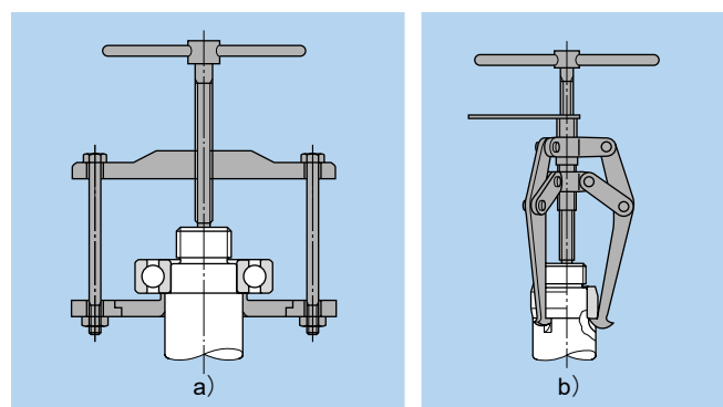
Fig.15.15 Desmontagem com extrator
