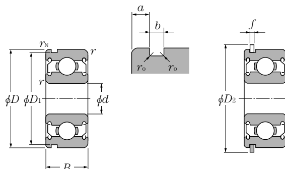
Ranhura para anel elástico Tipo blindado (ZZ)
