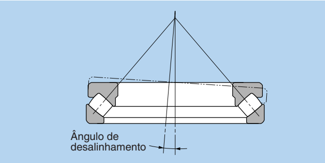
Fig. 2. Rolamento axial autocompensador de rolos
