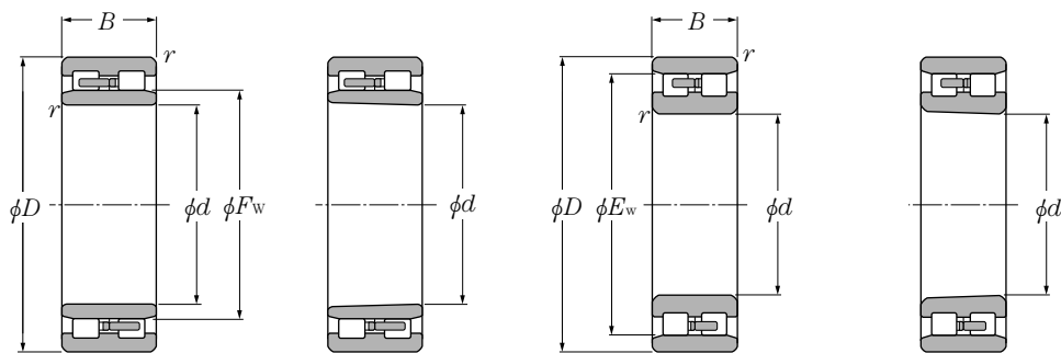
Tipo NNU Tipo NN Furo cilíndrico Furo cônico Furo cilíndrico Furo cônico
