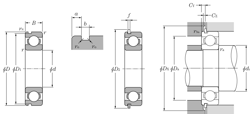
Com ranhura para anel elástico
