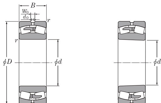
Furo cilíndrico
