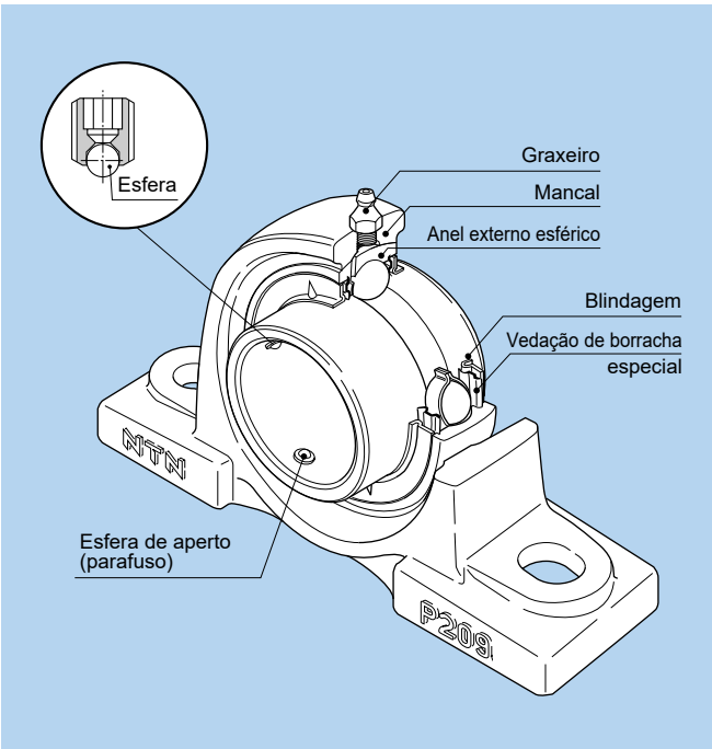
Fig. 1.4 Unidade de rolamento com graxeiro
