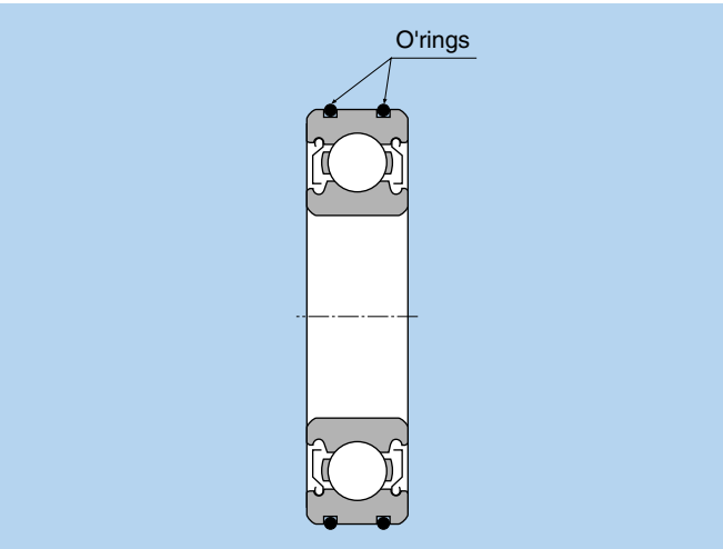
Fig. 3. Rolamento AC
