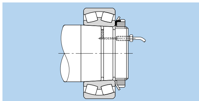
Fig. 15.8 Instalação utilizando injeção de óleo
