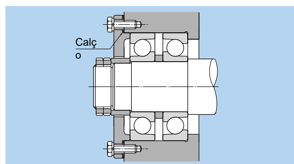
Fig. 15.14 Ajuste da folga interna axial utilizando calços
