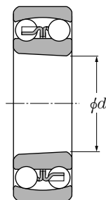
Furo cônico
