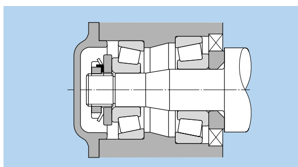
Fig. 15.12 Ajuste da folga interna axial
