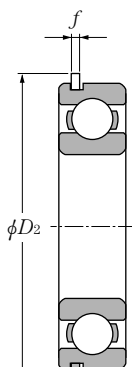
Com anel elástico
