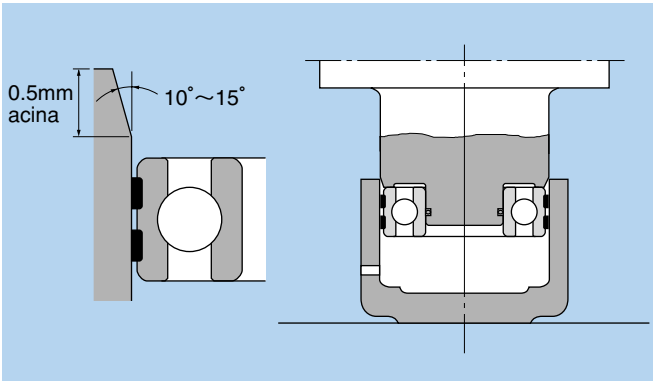
Fig. 2. Método de ajuste e chanfro do diâmetro interno do alojamento
