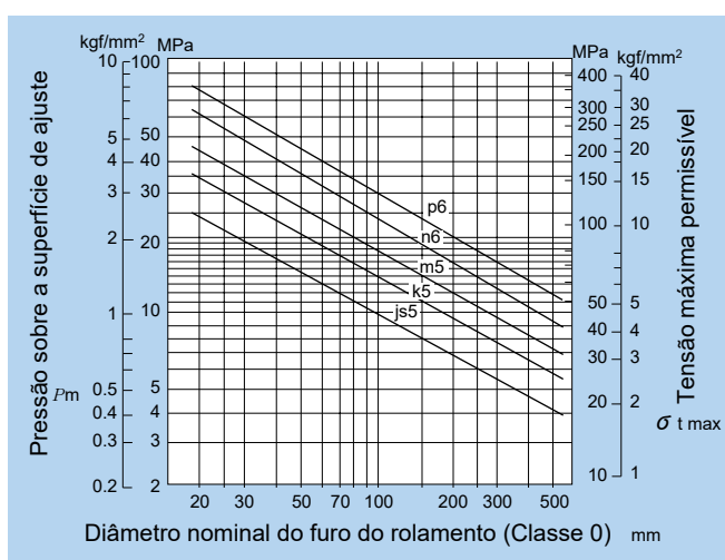
Fig.17.5.2 Interferência máxima de ajuste em relação à pressão da superfície ( P_m ) e à tensão máxima permissível ( \sigma_{t \max} )
