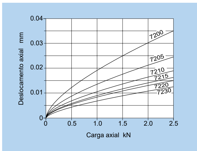
Fig.17.2.4 Carga axial e deslocamento axial da série 72
