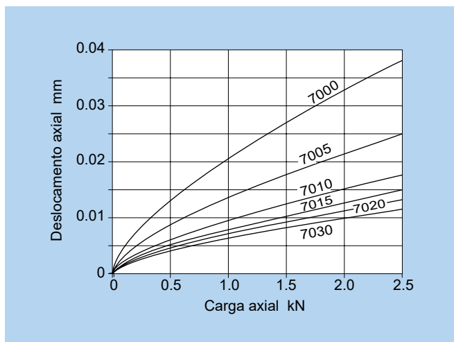
Fig. 17.2.2 Carga axial e deslocamento axial da série 70
