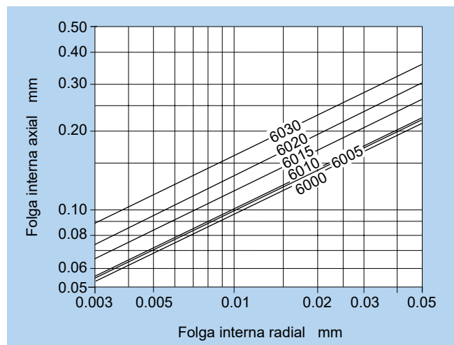
Fig. 17.1.3 Folga radial interna e axial da série 60
