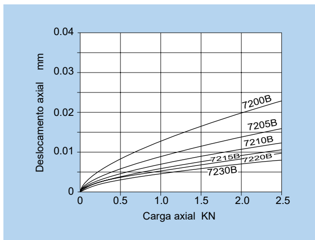
Fig. 17.2.5 Carga axial e deslocamento axial da série 72 B
