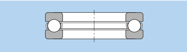
Fig. 1. Rolamento axial de esferas de escora simples (com gaiola prensada)
