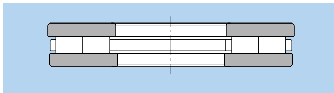
Fig. 3. Rolamento axial de dupla carreira de rolos cilíndricos
