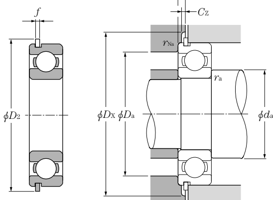
Com anel elástico
