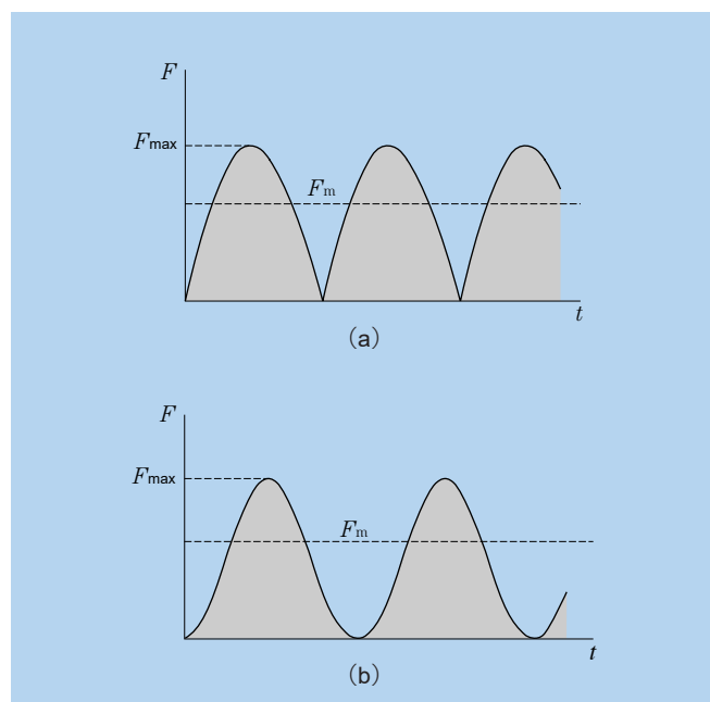
Fig. 4.11 Carga variável senoidal
