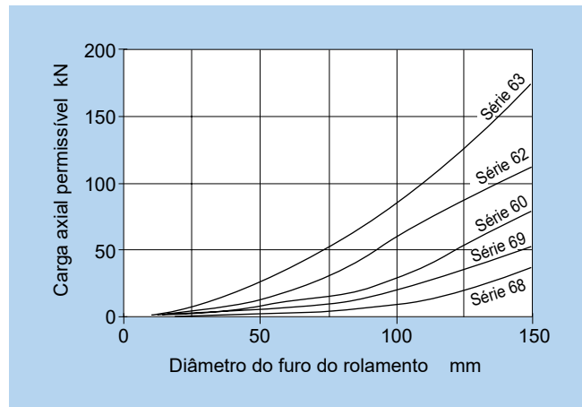
Fig. 17.4.1 Carga axial permissível para rolamentos rígidos de esferas
