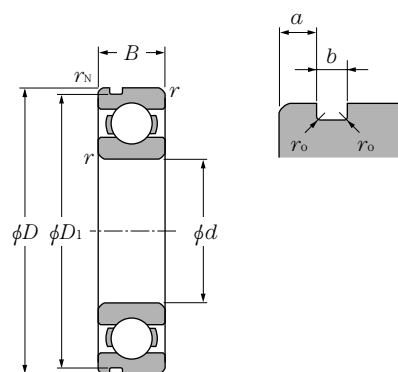
Com ranhura para anel elástico
