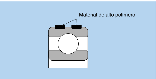
Fig. 1. Rolamentos com compensação de expansão
