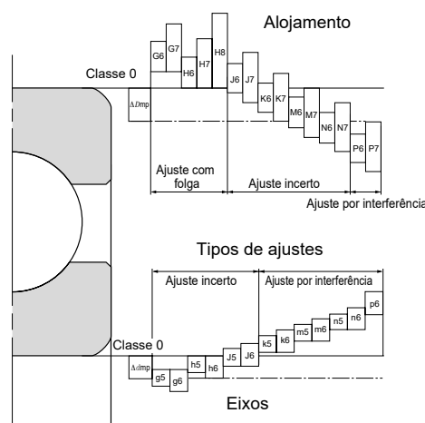
Fig 7.1 Ajustes
