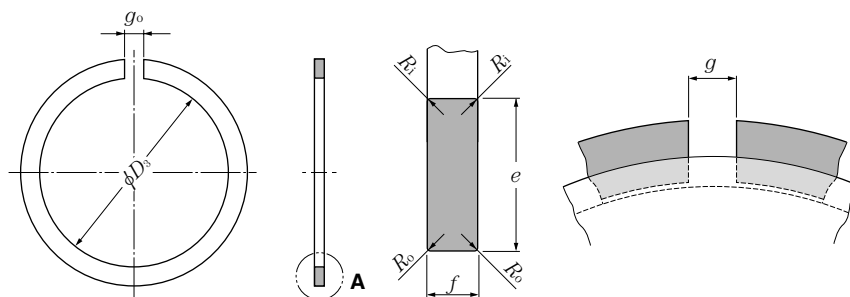
A (vista ampliada)
