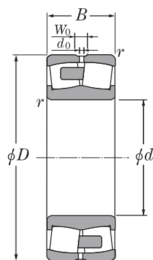
Furo cilíndrico tipo EM
