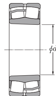
Furo cônico
