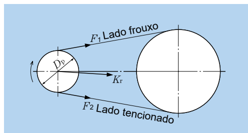
Fig. 4.6 Cargas em correntes / correias
