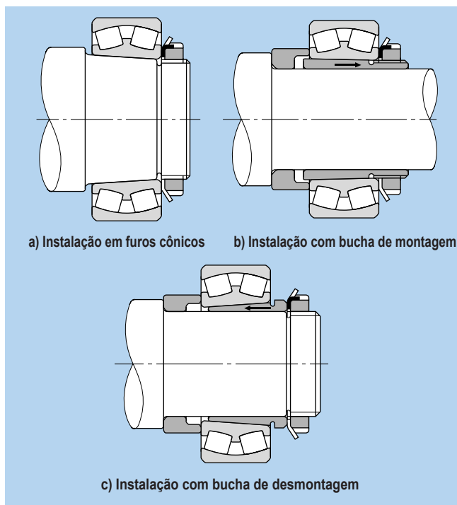
Fig. 15.7 Métodos de instalação utilizando porcas de fixação
