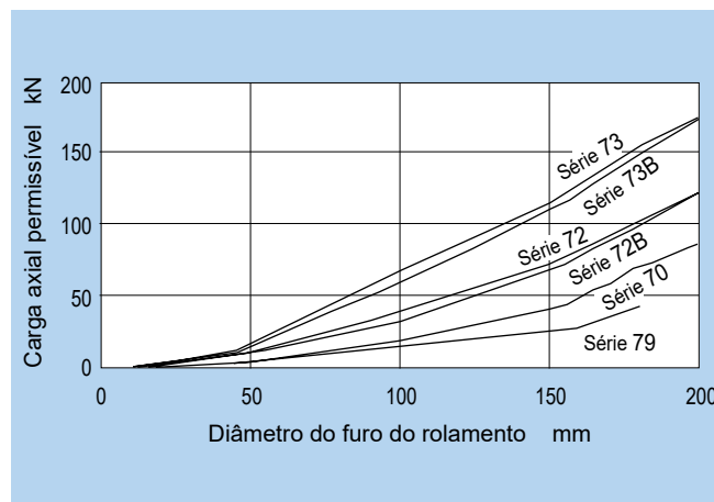
Fig. 17.4.2 Carga axial permissível para rolamentos de esferas de contato angular
