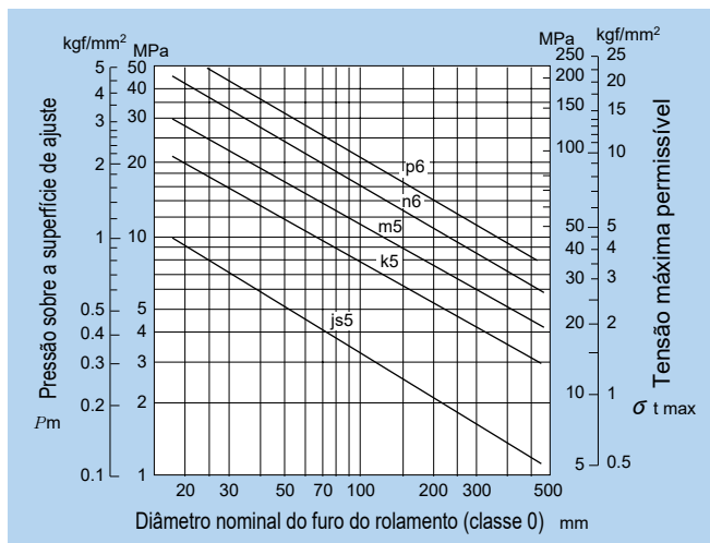
Fig.17.5.1 Interferência média de ajuste em relação à pressão da superfície ( P_m ) e à tensão máxima permissível ( \sigma_{t \max} )
