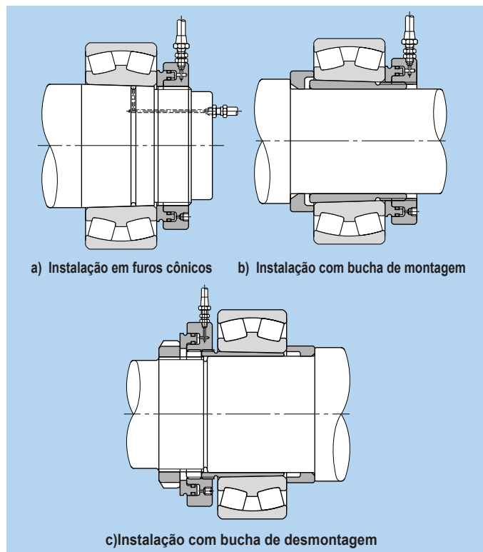
Fig. 15.9 Instalação utilizando uma porca hidráulica
