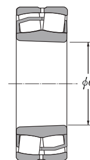
Furo cônico
