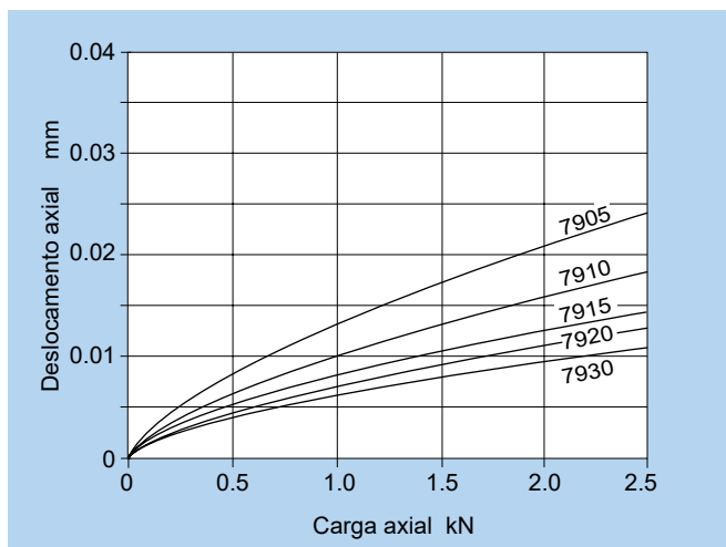
Fig. 17.2.1 Carga axial e deslocamento axial da série 79
