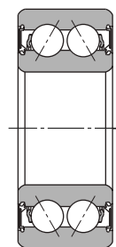
Vedação com contato (LLU)
