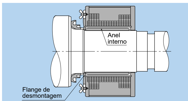
Fig. 15.6 Desmontagem de um anel interno utilizando um aquecedor por indução
