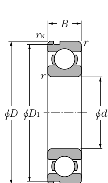
Com ranhura para anel elástico
