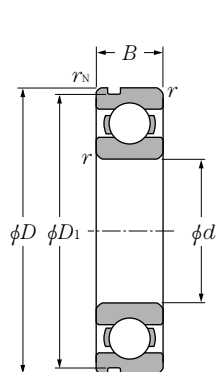
Com ranhura para anel elástico
