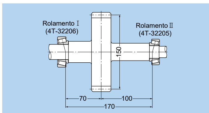
Fig. 4.13 Diagrama da engrenagem de dentes retos
