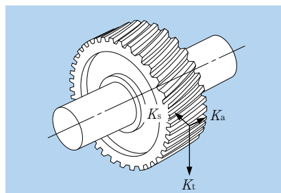
Fig. 4.2 Cargas de engrenagens helicoidais
