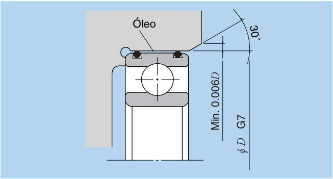
Fig. 4. Alojamento
