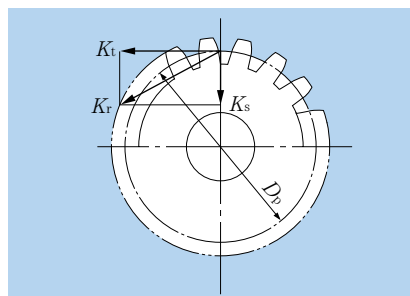
Fig. 4.3 Força radial resultante
